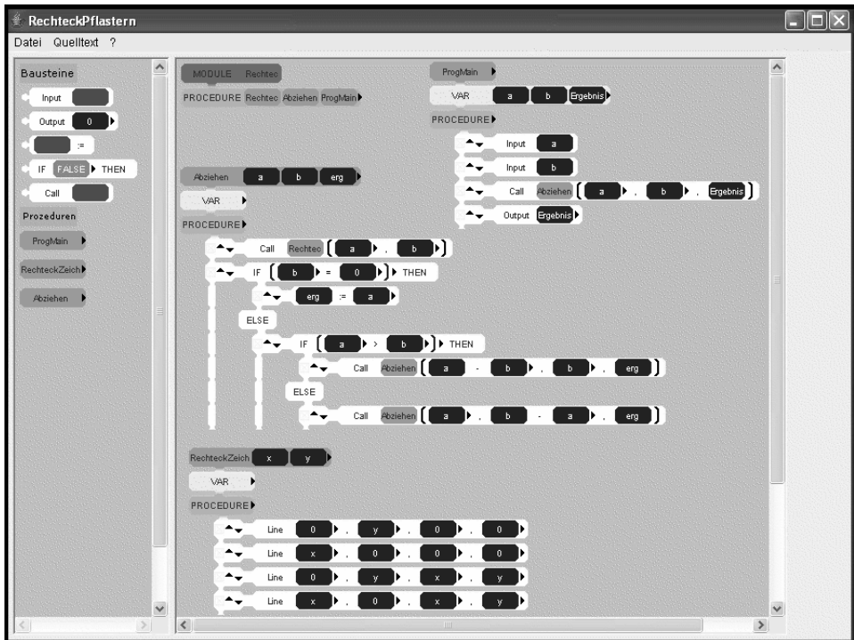
Abbildung 2: Das Programm zum Pflastern eines Rechteckes
