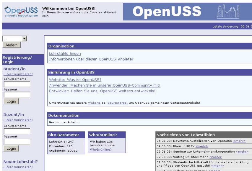
Abbildung 5: Das OpenUSS-Portal
