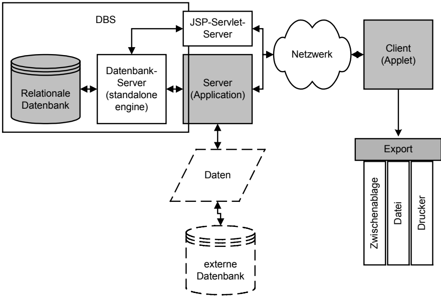
Abbildung 7: Systemarchitektur der Datenbank
