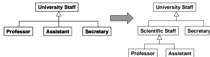
Abb. 2: Restrukturierung einer Klassenhierarchie als korrektkeiterhaltendes Refactoring
