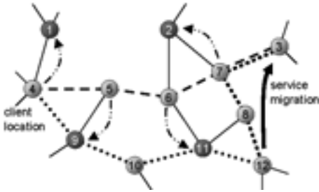
Abbildung 2: Anfrage-getriebene LS-Updates.
