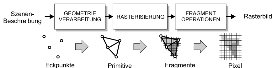
Abbildung 1: Die Graphik-Pipeline zum hardwarebeschleunigten Rendering.
